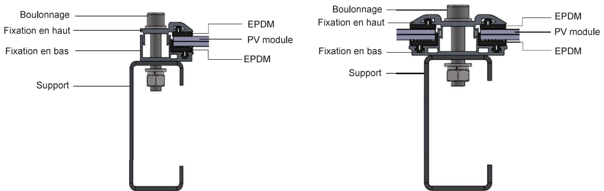
Double-face PV module de double verre (sans cadre)
