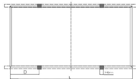
Installation avec la pièce de fixation (Longueur de pièce \geq 40\text{mm} )
