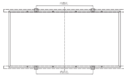
Installation par quatre trous intérieurs
