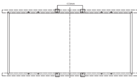
Installation à l'espace des trous de 400mm (La distance entre le côté C du cadre et le support pas moins de 30 mm)
