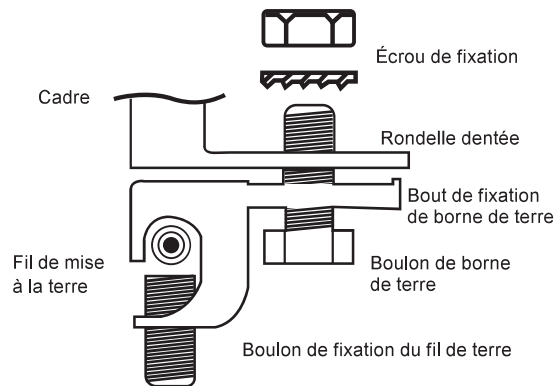
Figure 12 Méthode d'Installation
