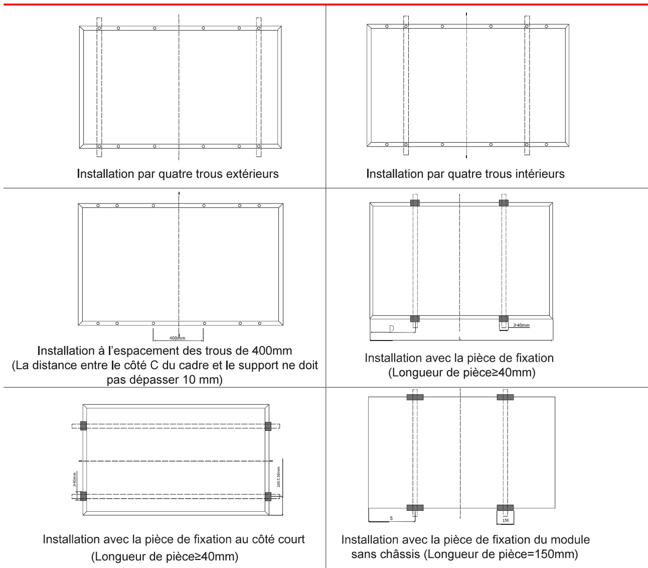
Figure 6 Icône d'installation du module monofacial
